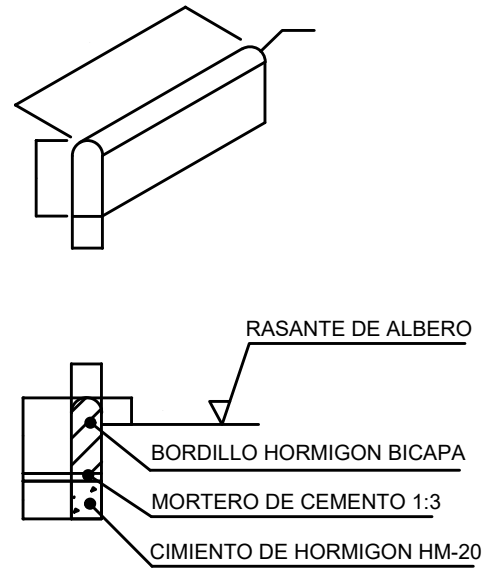
BORDILLO JARDIN DE HORMIGON BICAPA A4
