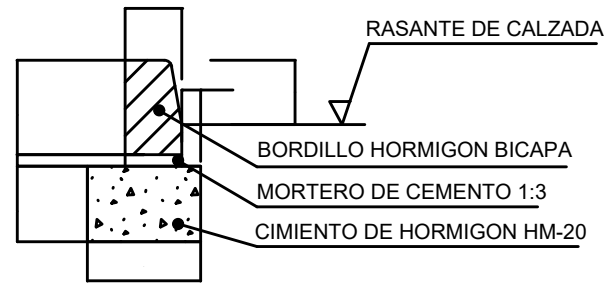
SECCION TIPO
