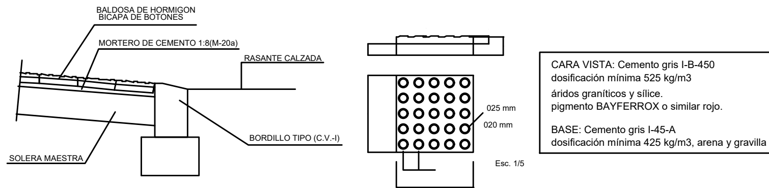
RAMPA EN PASO DE PEATONES
