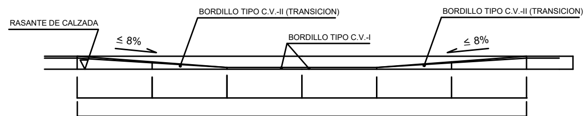
RAMPA EN PASO DE PEATONES
